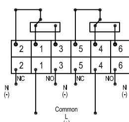
DIN PLUG
